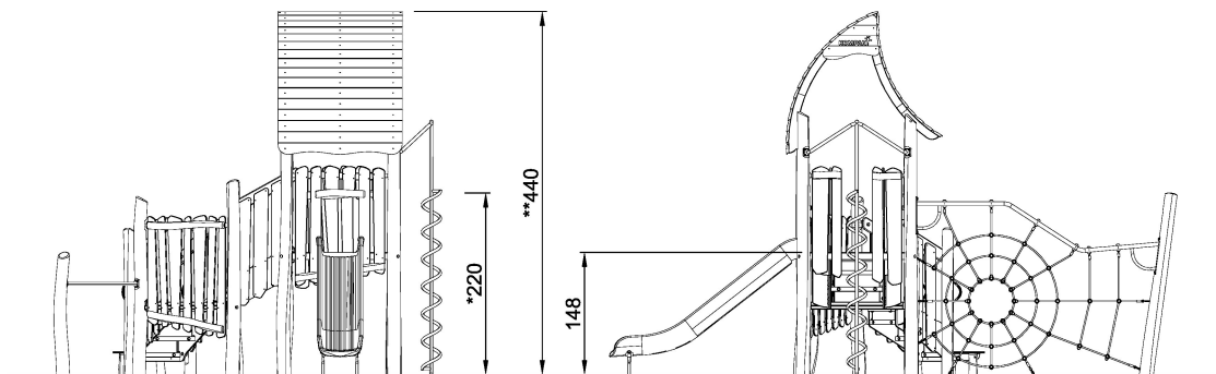
NRO2006 1:100
